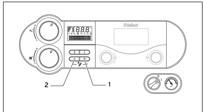
Abb. 4.18 Rauchfangkehrer-Betrieb einschalten (hier abgebildet: atmoTEC/turboTEC exclusiv)
