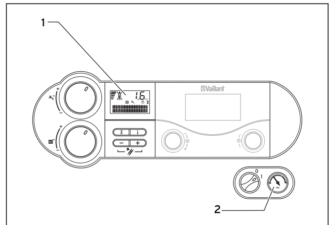
Abb. 4.16 Fülldruck der Heizungsanlage kontrollieren (hier abgebildet: atmoTEC/turboTEC exclusiv)
