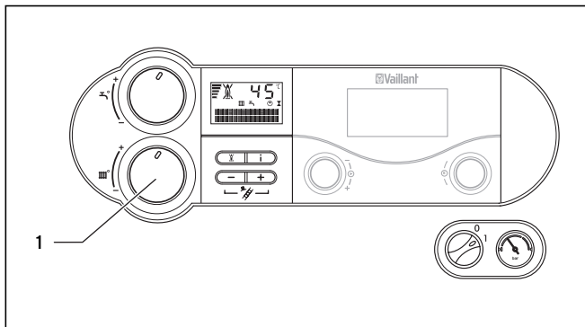
Abb. 4.11 Vorlauftemperatur-Einstellung mit angeschlossenem Regelgerät (hier abgebildet: atmoTEC/turboTEC exclusiv)
