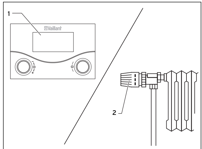
Abb. 4.13 Raumtemperaturregler/witterungsgeführte Regler einstellen
